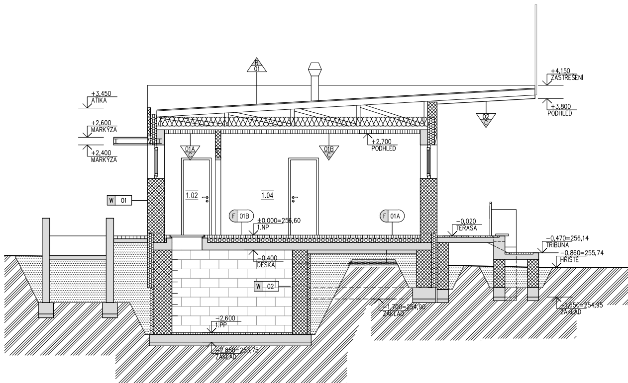
ŘEZ A-A
