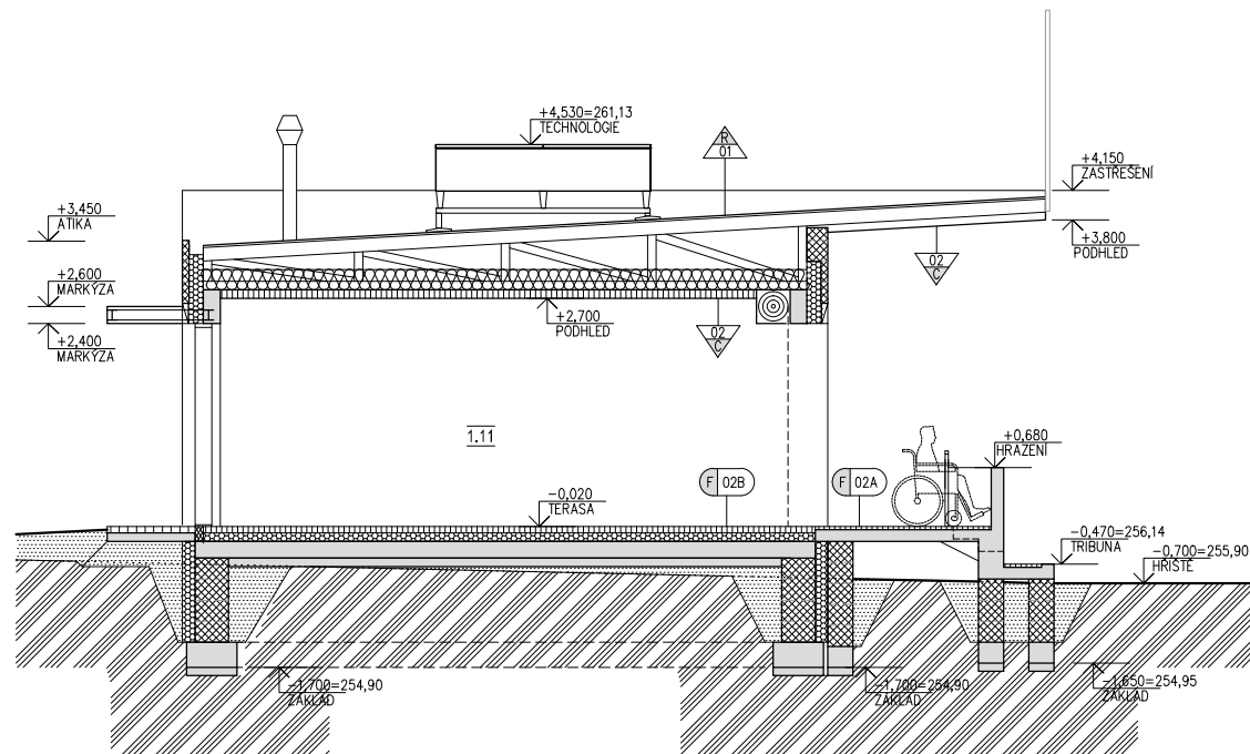
ŘEZ B-B
