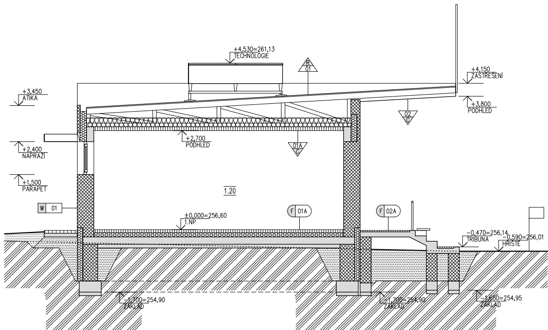
ŘEZ C-C
