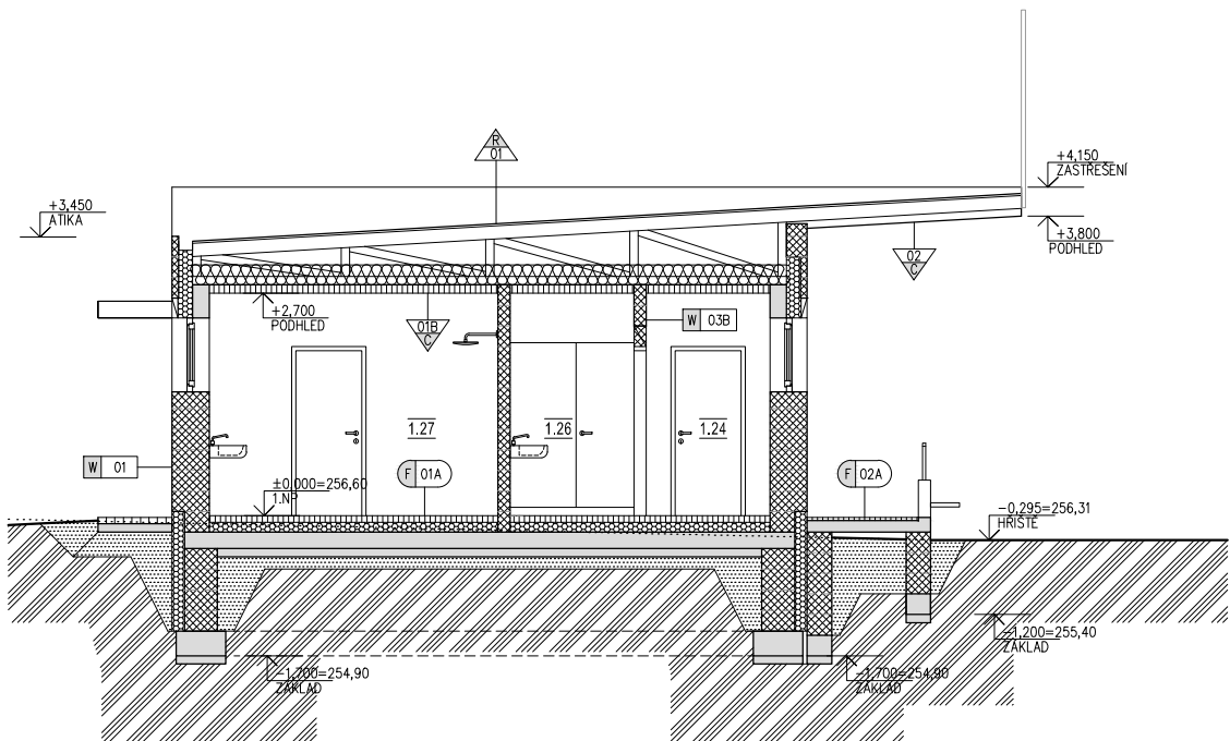
ŘEZ E-E
