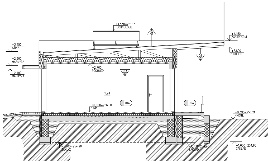
ŘEZ D-D
